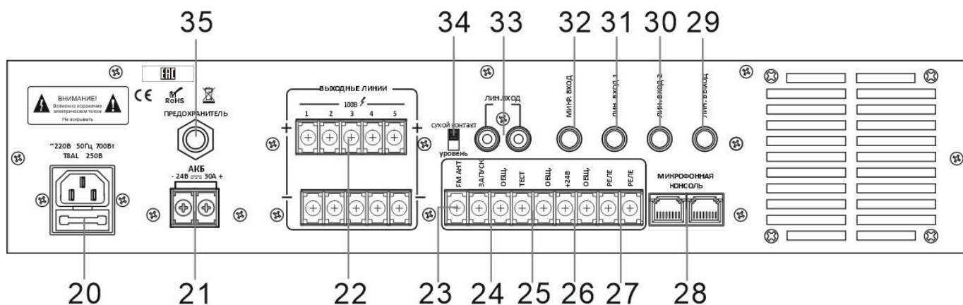
Рис. 1.3. Задняя панель
