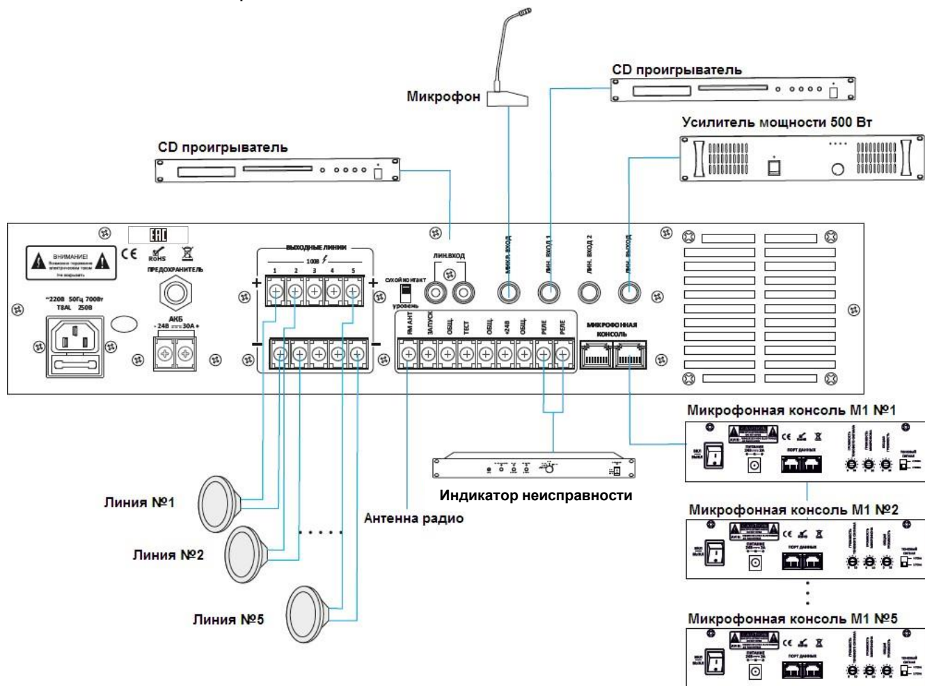
Рис. 2.1 Схема подключения
